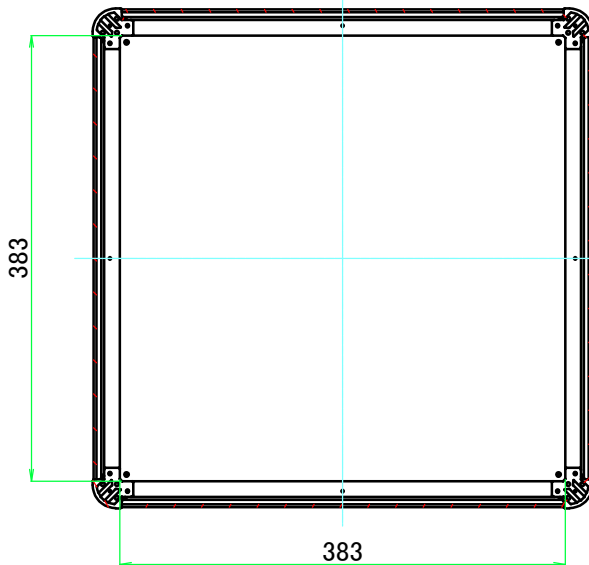
C-C ( 1 : 6.5 )
