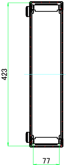
B-B ( 1 : 6.5 )
